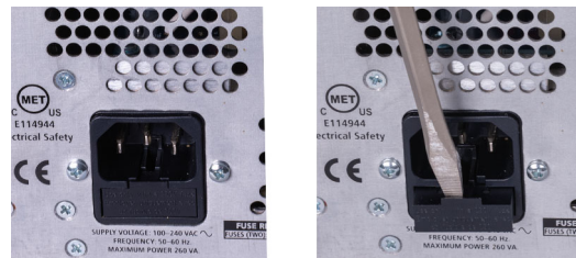
Module d'entrée d'alimentation Retrait du porte-fusibles
